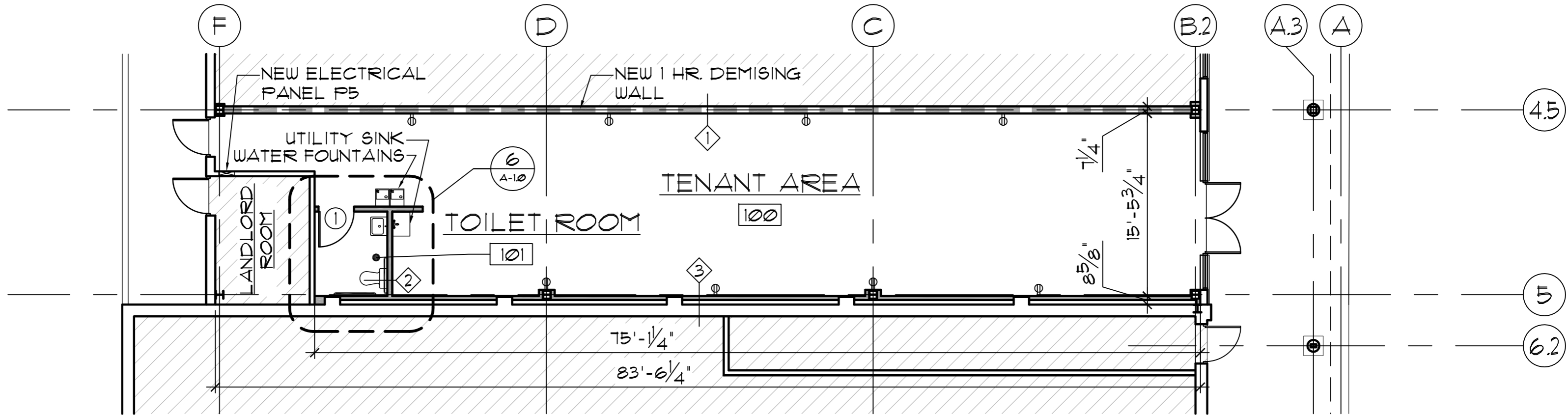
1 FLOOR PLAN SCALE: 1/8" = 1'-0"
